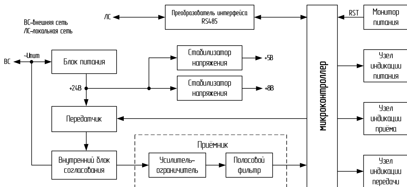
Рисунок 2. Структурная схема модуля связи НТС-7075-00
