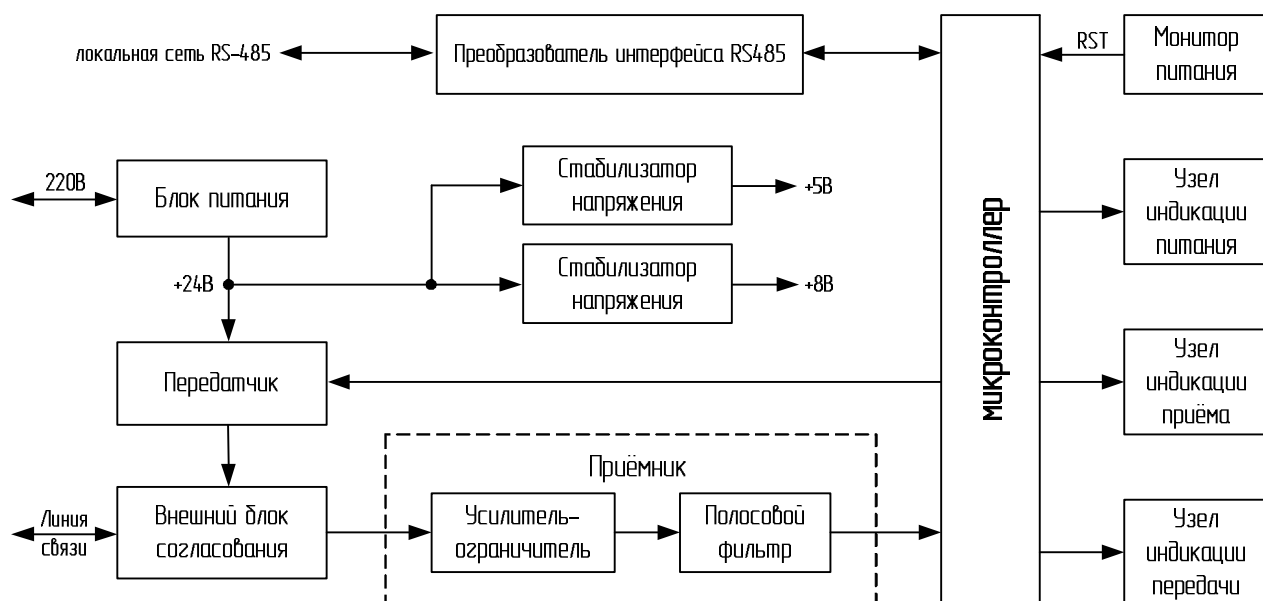
Рисунок 2. Структурная схема модуля связи НТС-7075-04
