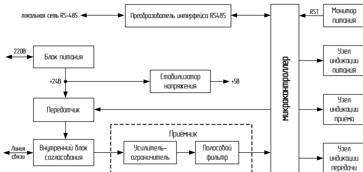
Рисунок 2. Структурная схема модуля связи НТС-7075-06
